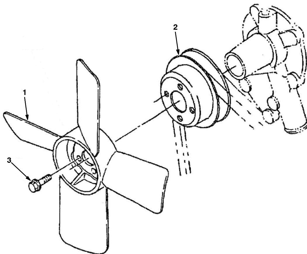
Fig. 22 - Fan Group
